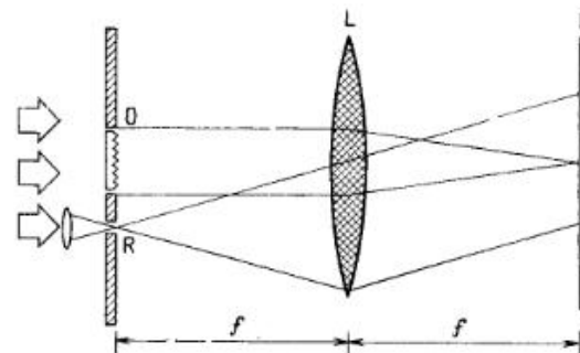
Рис. 6. Схема записи голограммы Фурье — Фраунгофера.
