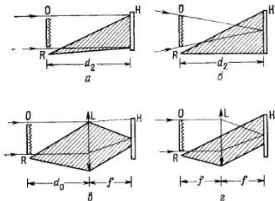
Рис. 3. Параметры эквивалентной безлинзовой голограммы Фурье для различных схем записи. a — безлинзовая голограмма Фурье (случай параллельного освещения), M = -1 , d_1 = \infty ; б — освещение сходящейся волной, M = -1 , d_1 = -d_2 ; в — объект перед линзой, d_1 = -d_2 = f[(d_0/f) - 1]^{-1} ; г — голограмма Фурье — Фраунгофера, d_1 = -d_2 = \infty , M/d_2 = -1/f .
