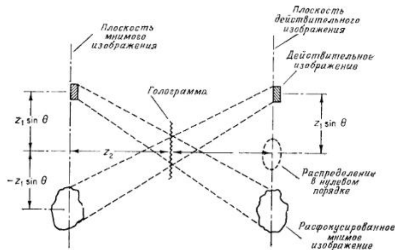
Рис. 3. Схематическое представление пространственного разделения сфокусированного действительного изображения от расфокусированного мнимого изображения и осевого распределения в случае объектов конечных размеров.
