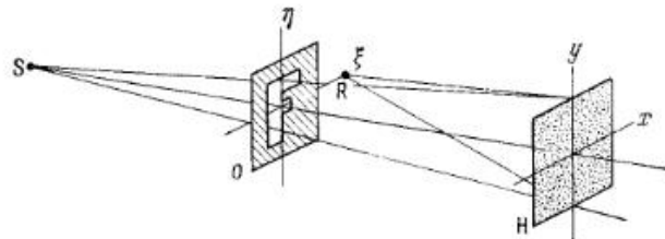
Рис. 1. Схема записи безлинзовой голограммы Фурье.
