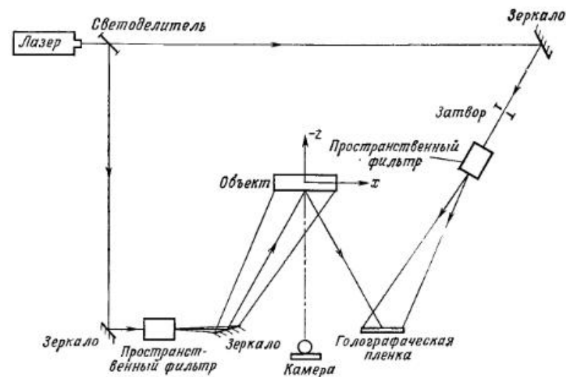
Рис. 12. Использование метода голографической спекл-интерферометрии в системе КМГНК.
