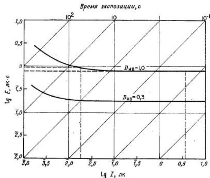
Рис. 12. Кривые нелинейности для типичной эмульсии.
