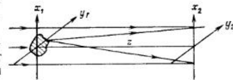
Рис. 1. Схематическое представление формирования голограммы Фраунгофера.
