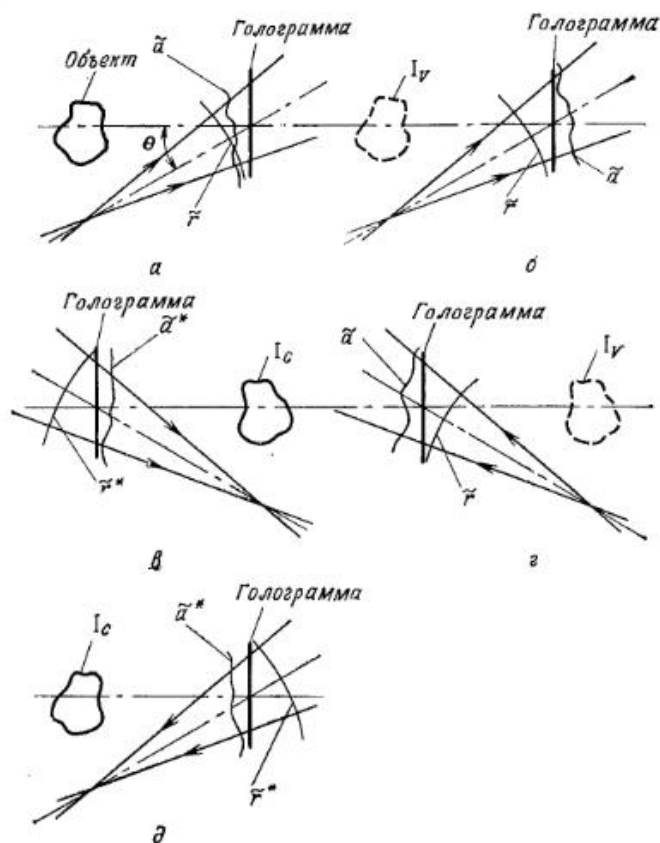
Рис. 2. Запись тонкой голограммы и восстановление с нее неискаженного изображения. I_c — сопряженное изображение; I_v — мнимое изображение; \vec{a} = a(x, y) \times \exp[i\varphi(x, y)] , \vec{a}^* = a(x, y) \exp[-i\varphi(x, y)] , \vec{r} = r \exp[i(bx + cx^2 + cy^2)] и \vec{r}^* = r \exp[-i(bx + cx^2 + cy^2)] .
