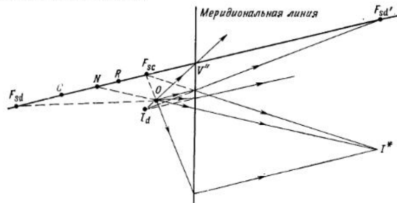
Рис. 6. Кардинальные точки голограммы и связанные с ними лучи (при получении изображений по типу IV и V).
