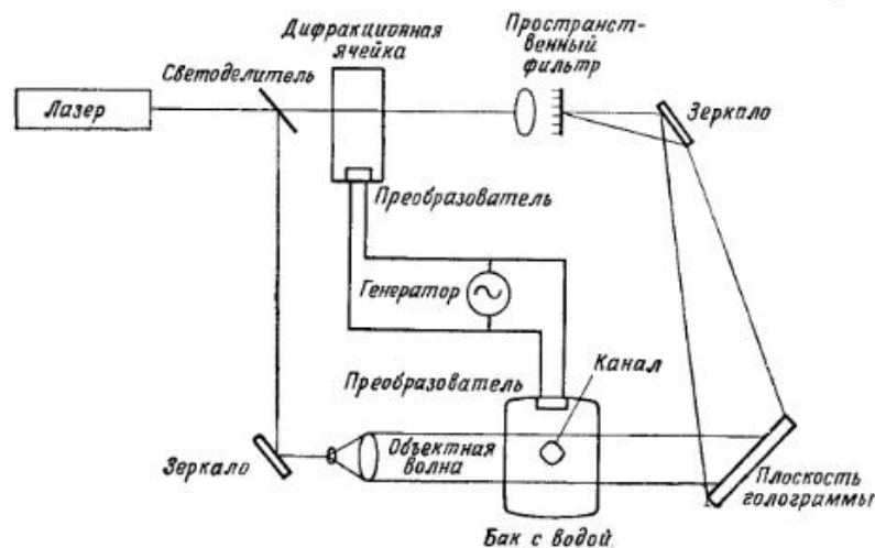
Рис. 20. Установка для получения голограмм ультразвуковых пучков.
