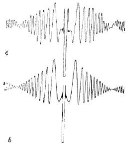
Рис. 3. Действительное изображение, формируемое показанной на рис. 2 голограммой Фраунгофера проволоки. a — позитивный отпечаток записи в плоскости сфокусированного изображения; b — микроденситограмма сечения негатива зарегистрированного изображения; a — теоретическая кривая. Согласно [7].
