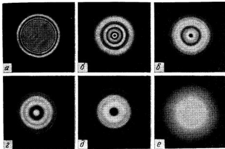
Рис. 8. Картины дифракции Френеля на круглой апертуре; величина z_0 остается постоянной, а z постепенно увеличивается от фото а к фото е.
