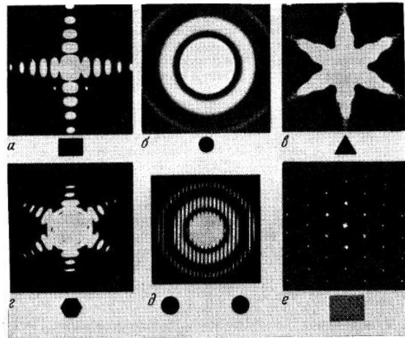
Рис. 9. Картины дифракции Фраунгофера на некоторых апертурах, показанных под каждым фото.
