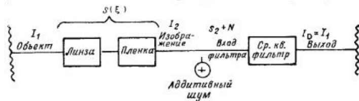
Рис. 8. Блок-схема системы формирования изображения в винеровской фильтрации.
