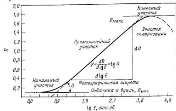
Рис. 2. Характеристическая кривая.
