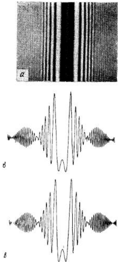
Рис. 2. Голограмма Фраунгофера проволоки диаметром 2a=100 мкм, полученная на расстоянии z=60 см от объекта при использовании света с длиной волны 514,6 нм. а — позитивный отпечаток части голограммы; б — микроденситограмма сечения голограммы; в — кривая, вычисленная на ЭВМ по формуле (6). Согласно [7].
