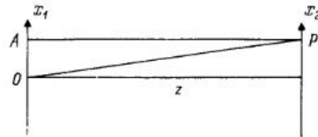
Рис. 4. Схема, используемая при пояснении требований к пространственной и временной когерентности освещения.
