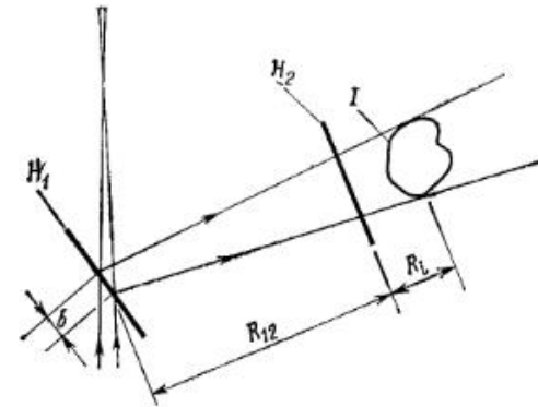
Рис. 8. Схема записи радужных голограмм. H_1 — исходная голограмма, с которой делается копия H_2 . Голограмма H_1 освещается через щель шириной b и длиной, равной длине голограммы.
