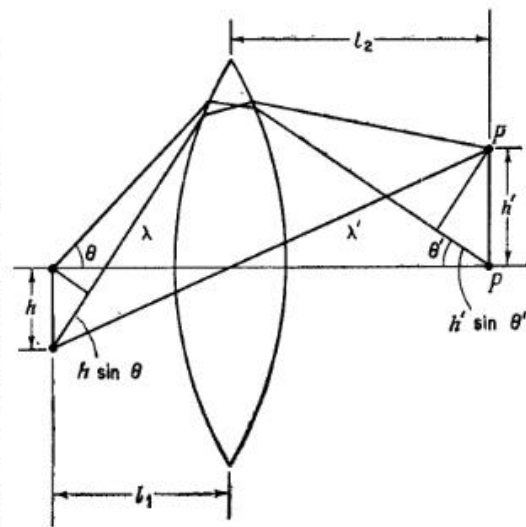
Рис. 5. К иллюстрации условия синусов Аббе.
