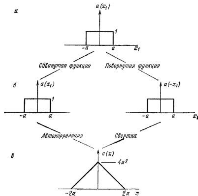
Рис. 4. Сравнение свертки и автокорреляции симметричных функций. а — симметричная прямоугольная функция; б — симметричные сдвинутая и повернутая функции; в — результирующая треугольная функция.
