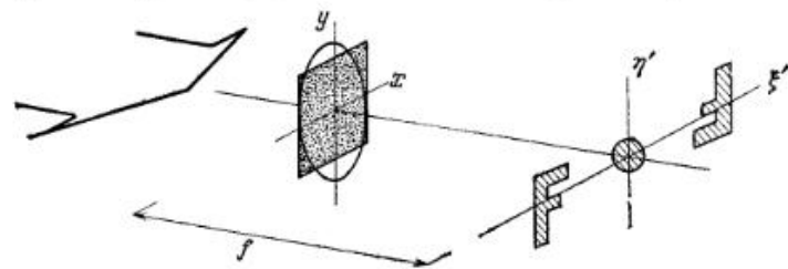
Рис. 4. Восстановление действительных изображений с голограммы Фурье.
