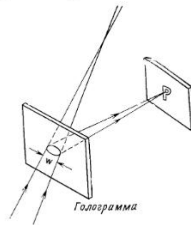
Рис. 5. Проекция восстановленного с голограммы изображения на экран с помощью лазерного пучка малого диаметра w .
