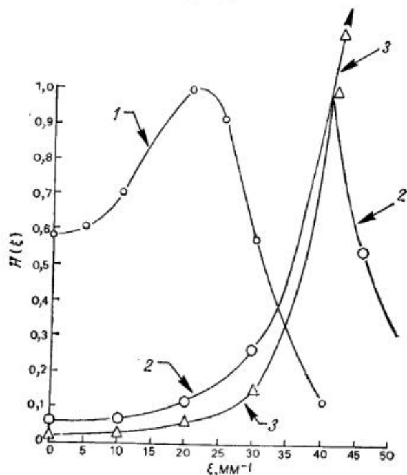
Рис. 9. Расчетные передаточные характеристики винеровских фильтров при различных значениях отношения сигнал/шум [C_{I,I_1}(\xi)/C_{NN}(\xi)] : кривая 1—10; кривая 2 — 100; кривая 3 — бесконечность. (Согласно Хорнеру [9].)
