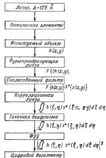
Рис. 15. Блок-схема голографической корреляционной установки. (Согласно Лиу и Оуэну [41].)
