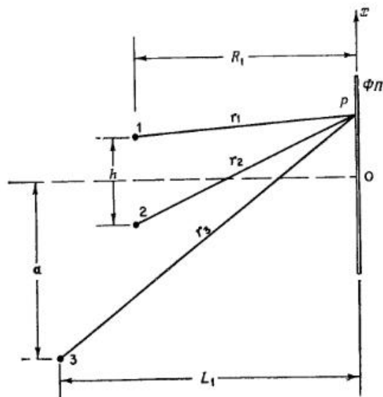
Рис. 6. Схема записи голограммы при определении поперечного увеличения. 1 и 2 — точечные объекты; 3 — точечный опорный источник; ФП — фотоэмульсия.
