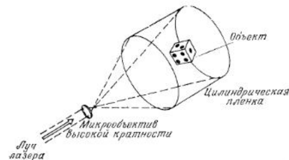
Рис. 2. Схема получения цилиндрической голограммы [6].
