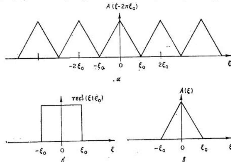
Рис. 2. Графическое представление теоремы выборки в частотной области. Произведение спектра A(\xi - 2n\xi_0) выборочной функции (а) и спектра интерполяционной функции (б) дает спектр A(\xi) (а).
