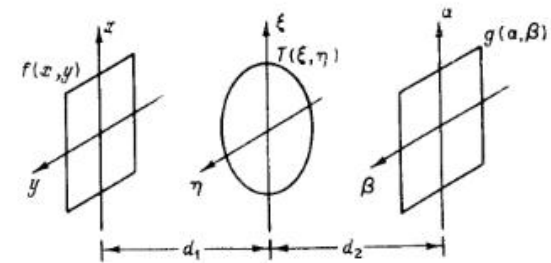
Рис. 2. Схема простой системы формирования изображения.
