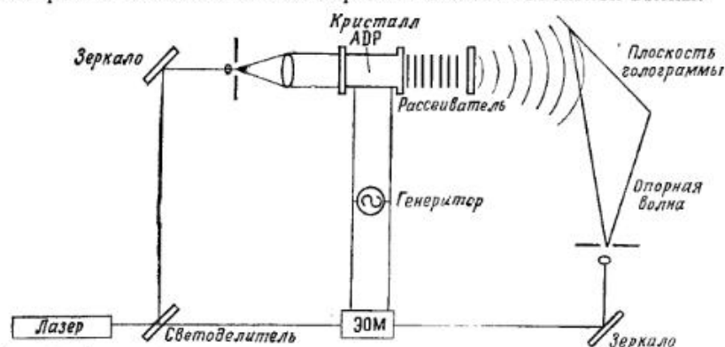
Рис. 22. Голографическая установка для определения резонанса волны сдвига в кристалле ADP.
