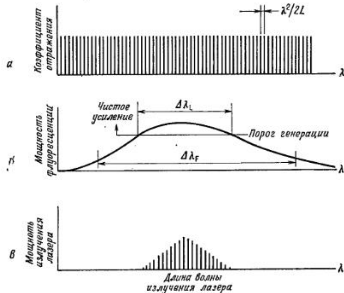
Рис. 2. Схематическое представление спектрального распределения мощности выходного излучения лазера без селекции мод. a — в оптическом резонаторе; b — в излучении флуоресценции активной среды; в — в выходном излучении лазера; \Delta\lambda_F — ширина спектра флуоресценции; \Delta\lambda_L — ширина спектра излучения лазера.
