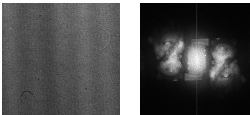
Рис. 2. – Высокоразрешающая цифровая голограмма размером 3.5 мм x 3.5мм отсканированная с разрешением. 2048x2048 (слева) и восстановленное из неё действительное и мнимое изображения (справа)
