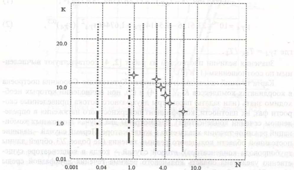
Рис. 2. Диаграмма режимов течения Кутателадзе–Сорокина:
