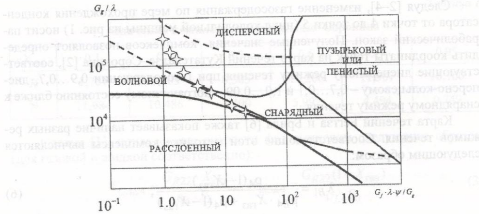
Рис. 3. Диаграмма Бейкера режимов горизонтального двухфазного двухкомпонентного потока (* — отмечены точки, соответствующие значениям из табл. 2)
